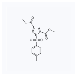
1059714 现货 CAS: 1191272-69-1
