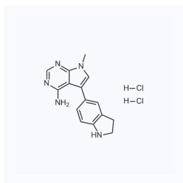
1182196 现货 CAS: 1337533-85-3
