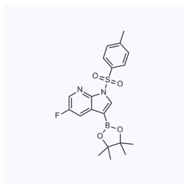
1127361 CAS: 1259279-57-6
