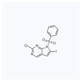
1127062 CAS: 1638760-67-4
