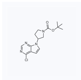
1112934 现货 CAS: 1240301-66-9
