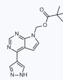
1125162 CAS: 1146629-77-7
