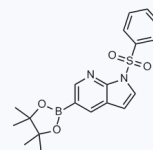
1066791 现货 CAS: 2058052-40-5
