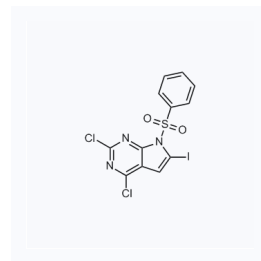
1127100 CAS: 1638763-86-6
