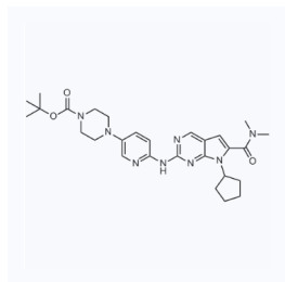
1079203 现货 CAS: 1374639-78-7
