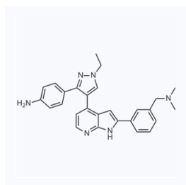
1075739 现货 CAS: 942919-53-1
