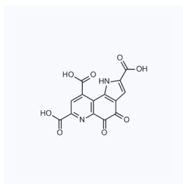
1040956 现货 CAS: 72909-34-3
