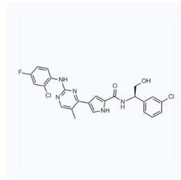
1077855 现货 CAS: 1680187-43-2
