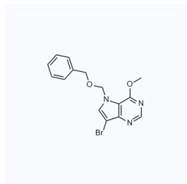
1061261 现货 CAS: 299916-62-4
