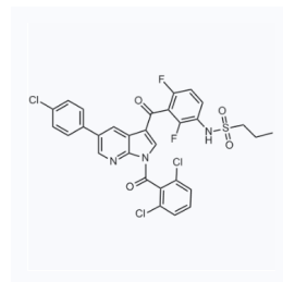
1057735 现货 CAS: 1262985-23-8
