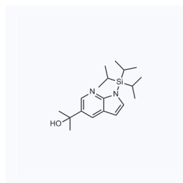
1048746 现货 CAS: 918523-63-4
