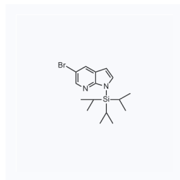
1048881 现货 CAS: 858116-66-2
