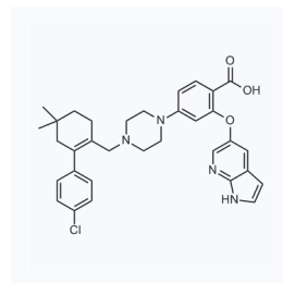
1080864 现货 CAS: 1235865-77-6
