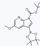
1127362 CAS: 1073338-94-9
