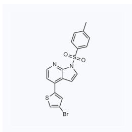
1058833 现货 CAS: 1415560-65-4
