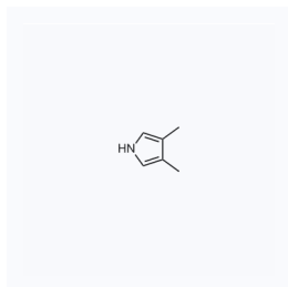
1122246 现货 CAS: 822-51-5
