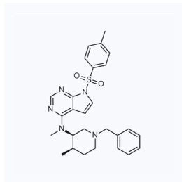
1060274 现货 CAS: 923036-30-0
