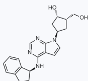
1058606 现货 CAS: 905580-90-7
