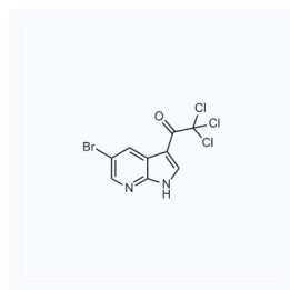
1048392 现货 CAS: 1379670-84-4
