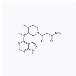
1060084 现货 CAS: 1675248-19-7
