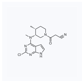
1060086 现货 CAS: 1616761-00-2
