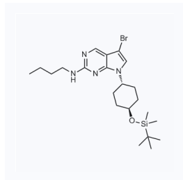
1061040 现货 CAS: 1429882-29-0
