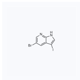
1042177 现货 CAS: 757978-18-0
