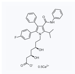
1076798 现货 CAS: 134523-03-8
