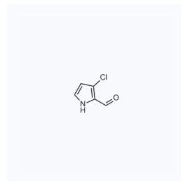
1125399 现货 CAS: 56164-42-2
