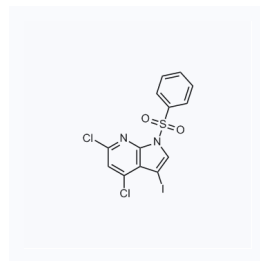
1123482 CAS: 2055841-50-2
