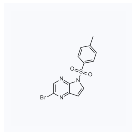
1063708 现货 CAS: 1201186-54-0
