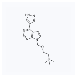
1049345 现货 CAS: 941685-27-4
