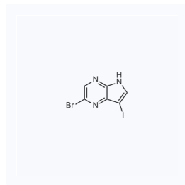
1089052 现货 CAS: 875781-44-5
