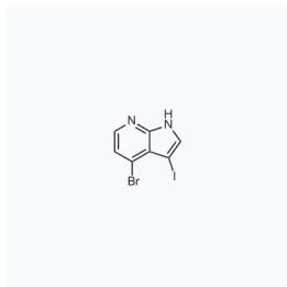
1064454 现货 CAS: 1000340-34-0
