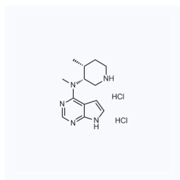
1060023 现货 CAS: 1655430-59-3
