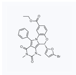
1111523 现货 CAS: 1415390-49-6
