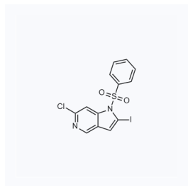
1123478 CAS: 1227267-17-5
