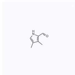
1122245 现货 CAS: 19713-89-4
