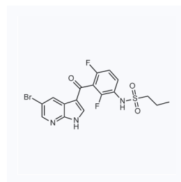
1057733 现货 CAS: 918504-27-5
