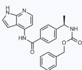
1058466 现货 CAS: 173897-93-3
