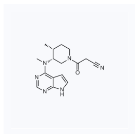
1070049 现货 CAS: 477600-75-2
