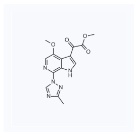
1059264 现货 CAS: 701214-00-8
