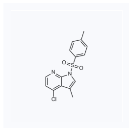
1058318 现货 CAS: 869335-18-2
