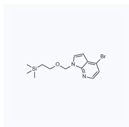
1074726 现货 CAS: 941685-08-1
