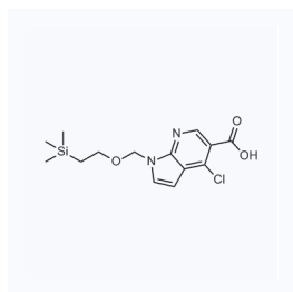
1074629 现货 CAS: 1039740-71-0
