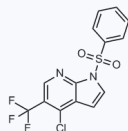
1058368 现货 CAS: 1196507-57-9
