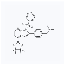
1058374 现货 CAS: 942919-72-4
