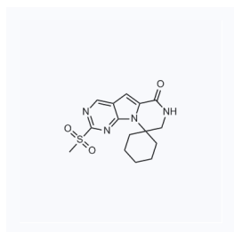
1135372 现货 CAS: 2170747-01-8
