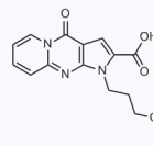
1146978 现货 CAS: 1086386-77-7
