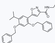
1057545 CAS: 747414-21-7
