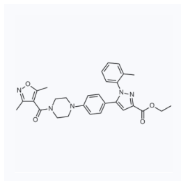
1058120 CAS: 1007477-05-5
