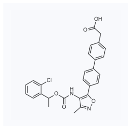
1059455 CAS: 1228689-85-7
