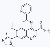
1059773 CAS: 1300737-69-2
