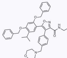
1057546 CAS: 747414-24-0
