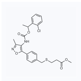
1030650 CAS: 355025-13-7
