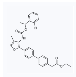
1059426 CAS: 1228690-21-8
