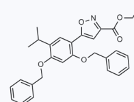
1057548 CAS: 747414-20-6
