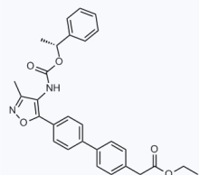
1059698 CAS: 1228690-38-7
