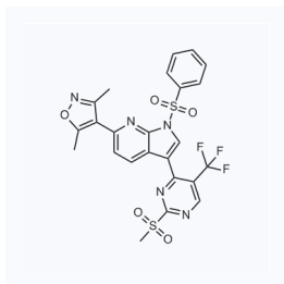
1176371 CAS: 2365230-38-0
