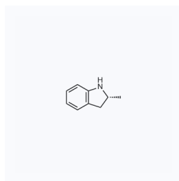
1124130 CAS: 22160-13-0
