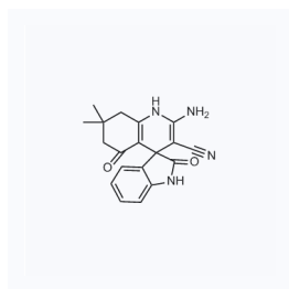
1143429 CAS: 314745-96-5
