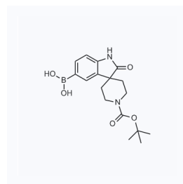
1109576 CAS: 1246372-96-2
