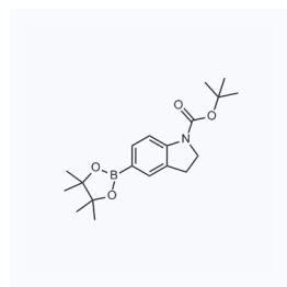
1044496 CAS: 837392-67-3
