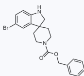
1108049 CAS: 438192-14-4
