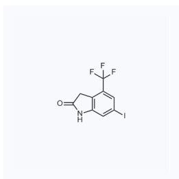
1165296 CAS: 259667-69-1
