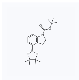
1111627 CAS: 1235451-62-3
