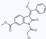
1060614 CAS: 1174335-83-1
