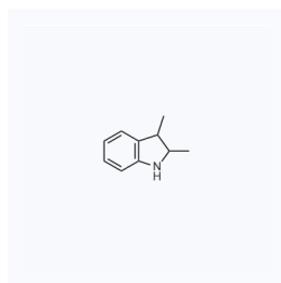
1207875 CAS: 22120-50-9
