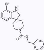
1108048 CAS: 1243461-51-9
