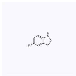
1026682 CAS: 2343-22-8
