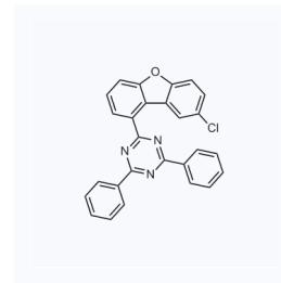
1182950 CAS: 2173554-85-1
