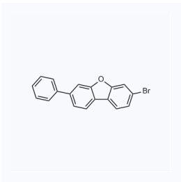
1178434 CAS: 2101813-26-5
