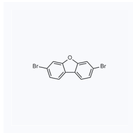
1178428 CAS: 67019-91-4
