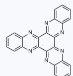
1181708 CAS: 214-83-5
