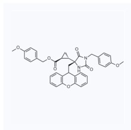
1059836 现货 CAS: 203209-15-8
