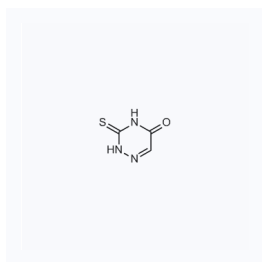
1201043 CAS: 626-08-4
