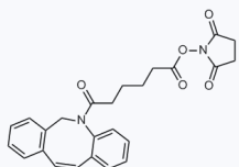
1158012 CAS: 1384870-47-6
