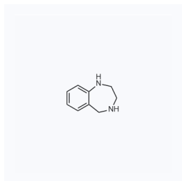
1197386 CAS: 5946-39-4
