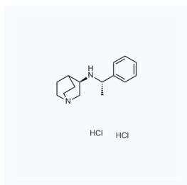
1049038 CAS: 120570-09-4
