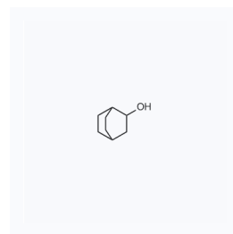
1162877 CAS: 18684-63-4
