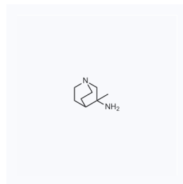
1171870 CAS: 21638-13-1
