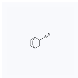
1162881 CAS: 6962-74-9
