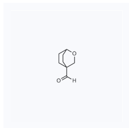
1122463 CAS: 1212021-23-2
