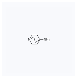
1162201 CAS: 22766-61-6
