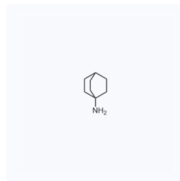
1124717 CAS: 1193-42-6
