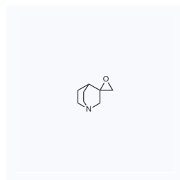
1057988 CAS: 41353-91-7
