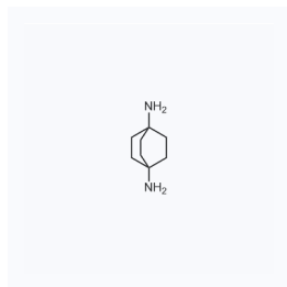
1124707 CAS: 1659-77-4
