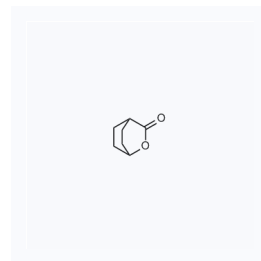
1172887 CAS: 4350-84-9
