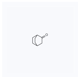
1065513 CAS: 2716-23-6
