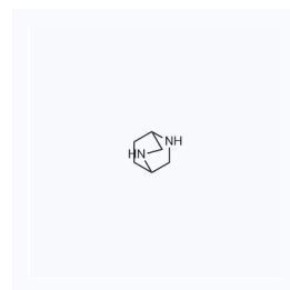
1177245 CAS: 658-24-2
