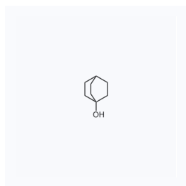
1120424 CAS: 20534-58-1
