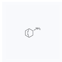
1191060 CAS: 130463-97-7
