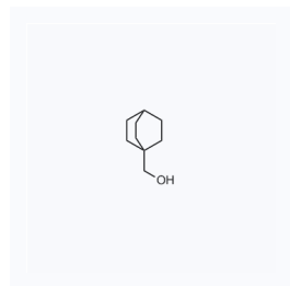
1123587 CAS: 2574-42-7
