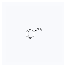
1071529 CAS: 123536-15-2
