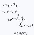
1037011 CAS: 5949-16-6
