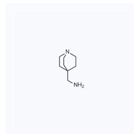
1069775 CAS: 67496-78-0
