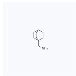
1162886 CAS: 25344-96-1
