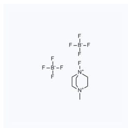
1066184 CAS: 159269-48-4
