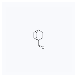
1182726 CAS: 2064-05-3
