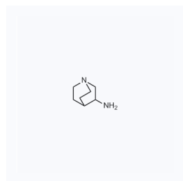
1171872 CAS: 6238-14-8
