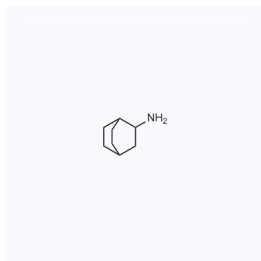
1162879 CAS: 20643-57-6
