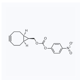
1155583 CAS: 1263166-91-1
