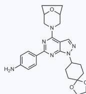
1058705 现货 CAS: 1144068-84-7
