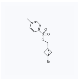
1149106 CAS: 137741-19-6
