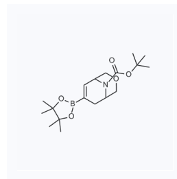
1126310 CAS: 1313034-29-5
