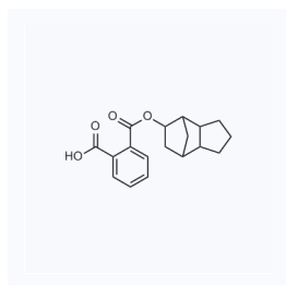
1058987 CAS: 109821-56-9
