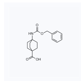
1121712 CAS: 444344-91-6
