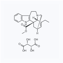
1056943 CAS: 4168-17-6
