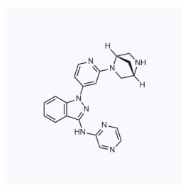
1125195 CAS: 1394066-99-9
