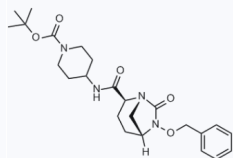
1061293 现货 CAS: 1174020-63-3
