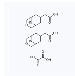
1120001 CAS: 1523530-64-4
