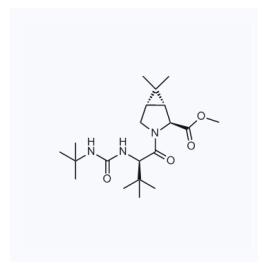
1060213 CAS: 2170811-36-4
