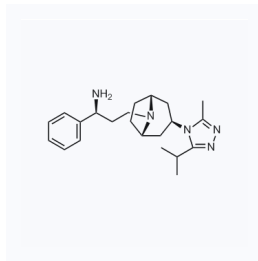
1051297 CAS: 376348-71-9
