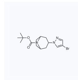
1092505 CAS: 1224194-51-7
