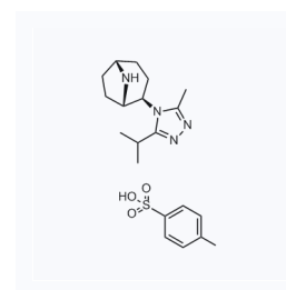
1051311 CAS: 423165-08-6
