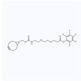
1185534 CAS: 1421932-53-7
