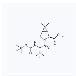
1060212 CAS: 394735-26-3
