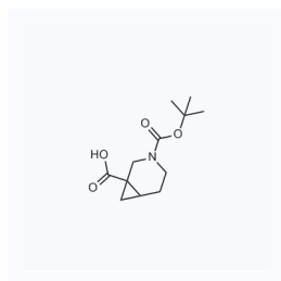
1148029 现货 CAS: 1239421-67-0
