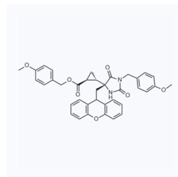
1059836 现货 CAS: 203209-15-8
