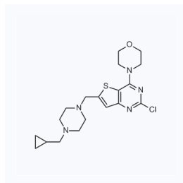
1060572 现货 CAS: 885699-88-7
