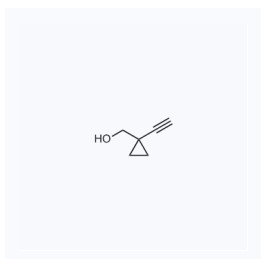
1124300 CAS: 871476-77-6
