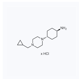
1057889 现货 CAS: 876371-19-6
