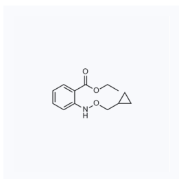
1170909 现货 CAS: 1616691-65-6
