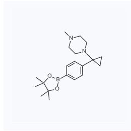
1123080 CAS: 1643923-77-6
