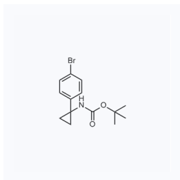
1111682 现货 CAS: 360773-84-8
