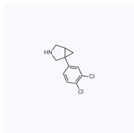
1123538 现货 CAS: 66504-40-3
