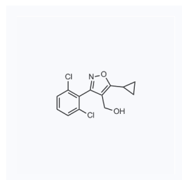
1183541 现货 CAS: 946426-89-7
