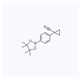
1108308 现货 CAS: 1206641-31-7
