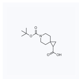
1052883 现货 CAS: 871727-05-8
