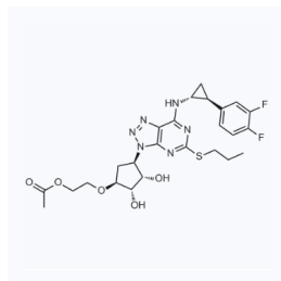
1080421 现货 CAS: 1616703-93-5
