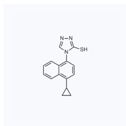
1061011 现货 CAS: 1533519-84-4
