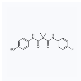
1061867 现货 CAS: 849217-60-3
