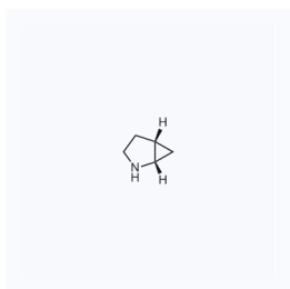
1128585 CAS: 842949-51-3
