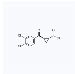
1099131 现货 CAS: 213400-32-9
