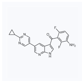
1061899 现货 CAS: 1859158-65-8
