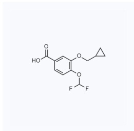
1062959 现货 CAS: 162401-62-9
