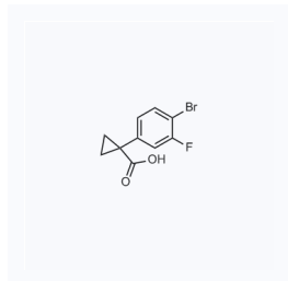
1125158 现货 CAS: 749269-74-7
