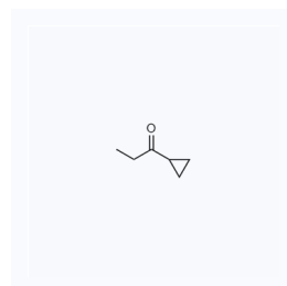
1123212 CAS: 6704-19-4
