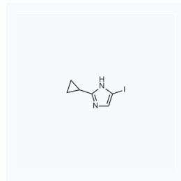
1112396 现货 CAS: 761426-65-7
