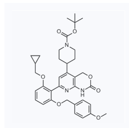
1059827 现货 CAS: 2444010-25-5
