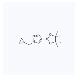
1064501 现货 CAS: 1000801-75-1
