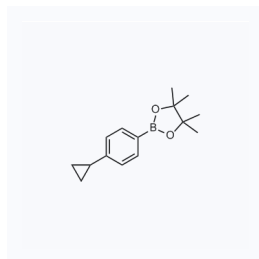
1113042 现货 CAS: 1219741-94-2
