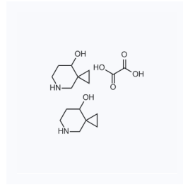
1172943 CAS: 2173093-13-3
