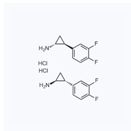
1059279 现货 CAS: 1156491-10-9
