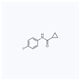
1115620 现货 CAS: 23779-17-1
