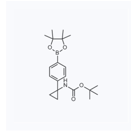
1171977 CAS: 1313441-88-1
