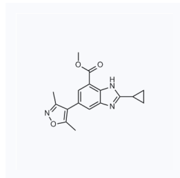
1176067 现货 CAS: 1637771-11-9
