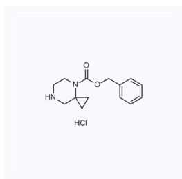
1060232 现货 CAS: 1951440-78-0
