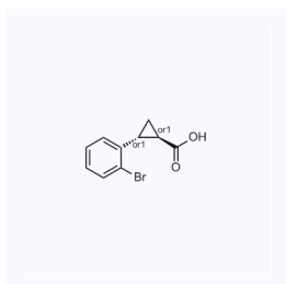
1115204 现货 CAS: 175168-70-4
