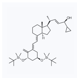
1058472 现货 CAS: 112849-27-1
