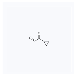
1159686 CAS: 5617-85-6
