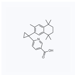
1022368 现货 CAS: 153559-76-3
