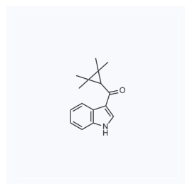
1159740 现货 CAS: 895152-66-6
