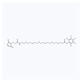
1186862 CAS: 1599432-34-4
