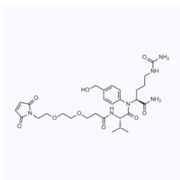
1176464 CAS: 2055041-38-6
