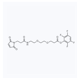
1176528 CAS: 1431291-44-9
