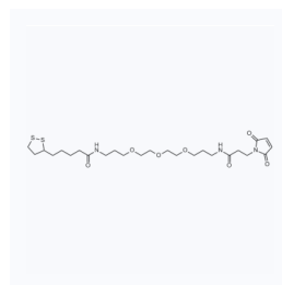
1185093 CAS: 1314378-19-2
