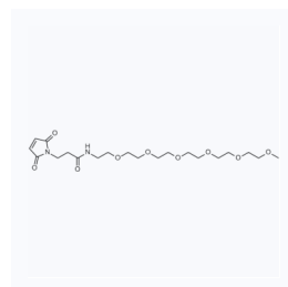
1175881 CAS: 1644231-07-1
