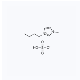
1027750 CAS: 262297-13-2
