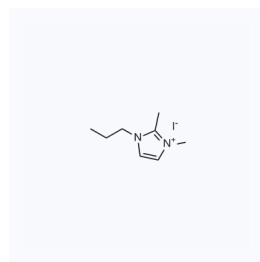
1026035 CAS: 218151-78-1
