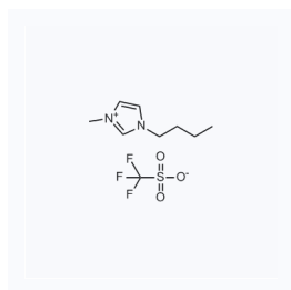
1023803 CAS: 174899-66-2
