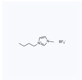
1023767 现货 CAS: 174501-65-6
