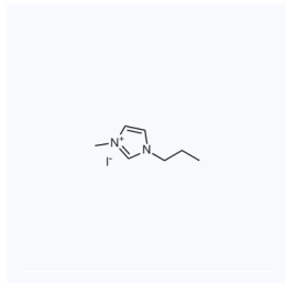
1017872 现货 CAS: 119171-18-5
