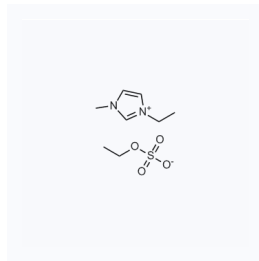
1030164 CAS: 342573-75-5
