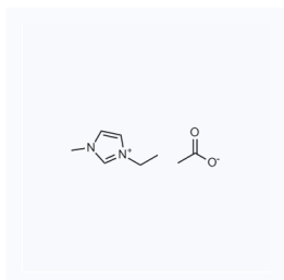
1021392 现货 CAS: 143314-17-4
