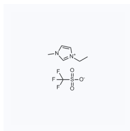
1021588 CAS: 145022-44-2
