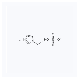
1032246 CAS: 412009-61-1
