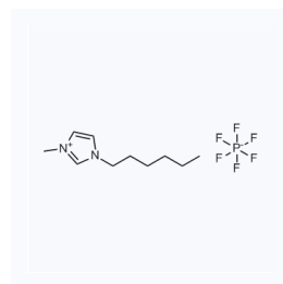
1028879 CAS: 304680-35-1
