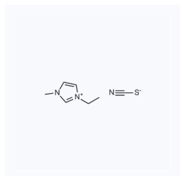
1029838 现货 CAS: 331717-63-6
