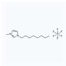
1028880 CAS: 304680-36-2
