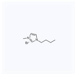
1044833 现货 CAS: 85100-77-2
