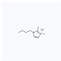
1047716 现货 CAS: 98892-75-2
