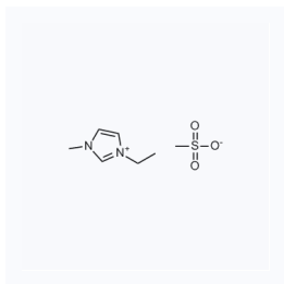
1021589 CAS: 145022-45-3
