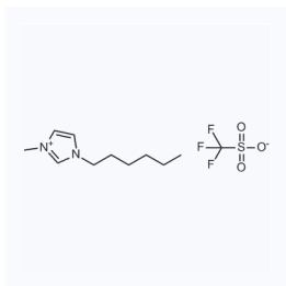
1033073 CAS: 460345-16-8
