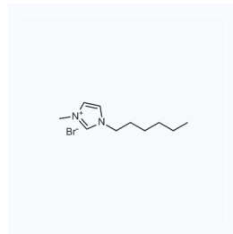
1044834 CAS: 85100-78-3
