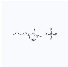
1032021 现货 CAS: 402846-78-0
