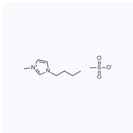
1030171 CAS: 342789-81-5
