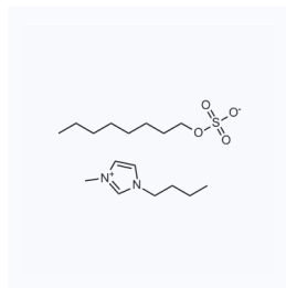
1032823 CAS: 445473-58-5
