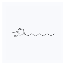
1037800 CAS: 61545-99-1
