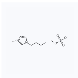
1031950 CAS: 401788-98-5
