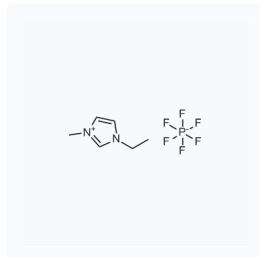
1022485 现货 CAS: 155371-19-0
