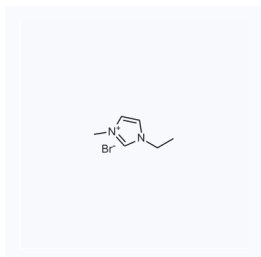
1039109 现货 CAS: 65039-08-9
