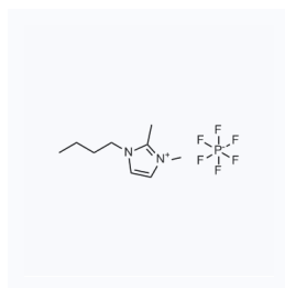
1026455 CAS: 227617-70-1
