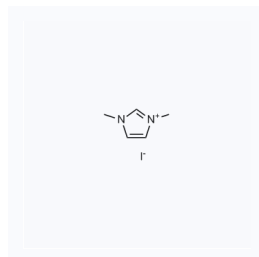
1109085 现货 CAS: 4333-62-4
