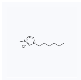
1023522 现货 CAS: 171058-17-6
