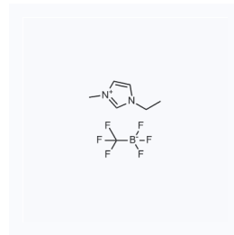
1039790 CAS: 681856-28-0
