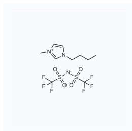
1023805 现货 CAS: 174899-83-3
