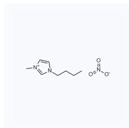
1024047 现货 CAS: 179075-88-8
