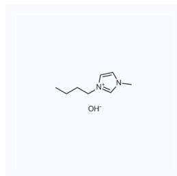
1172509 现货 CAS: 528818-81-7
