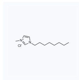
1039040 CAS: 64697-40-1
