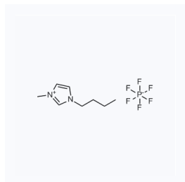
1023766 现货 CAS: 174501-64-5
