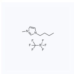
1041183 CAS: 741677-68-9
