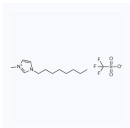
1032051 现货 CAS: 403842-84-2
