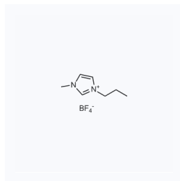
1158786 CAS: 244193-48-4
