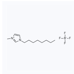
1027042 现货 CAS: 244193-52-0
