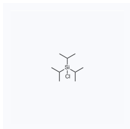
1062042 现货 CAS: 13154-24-0
