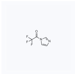
1022434 现货 CAS: 1546-79-8
