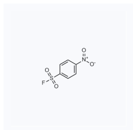
1030444 现货 CAS: 349-96-2
