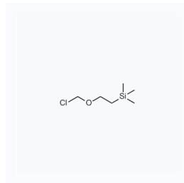
1042491 现货 CAS: 76513-69-4
