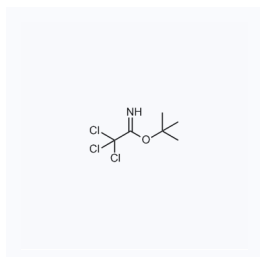
1047731 现货 CAS: 98946-18-0
