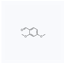
1066189 现货 CAS: 613-45-6
