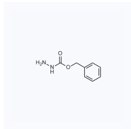
1034904 现货 CAS: 5331-43-1
