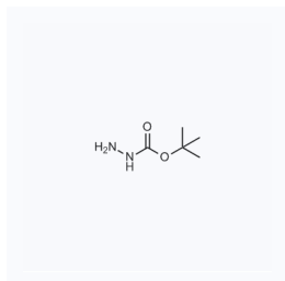
1045248 现货 CAS: 870-46-2
