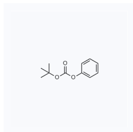
1039373 现货 CAS: 6627-89-0
