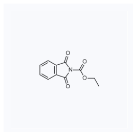
1083113 现货 CAS: 22509-74-6
