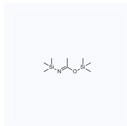
1015525 现货 CAS: 10416-59-8
