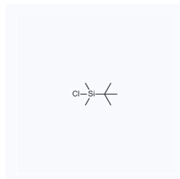
1024139 现货 CAS: 18162-48-6
