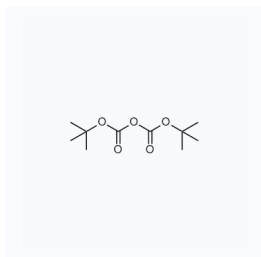
1027048 现货 CAS: 24424-99-5
