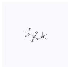
1083303 现货 CAS: 27607-77-8
