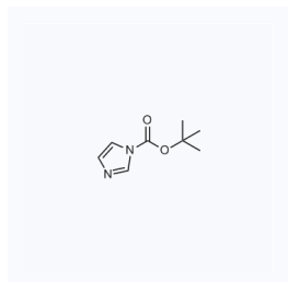
1033722 现货 CAS: 49761-82-2
