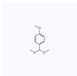
1026059 现货 CAS: 2186-92-7
