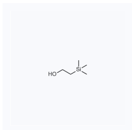
1028503 现货 CAS: 2916-68-9
