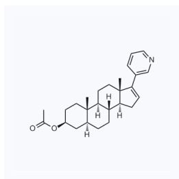
1060160 现货 CAS: 219843-76-2
