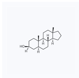
1018517 CAS: 1224-92-6
