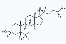
1028350 CAS: 2868-48-6
