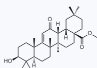
1057711 CAS: 65023-19-0
