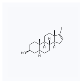
1060158 现货 CAS: 95043-81-5
