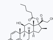
1025896 CAS: 2152-44-5
