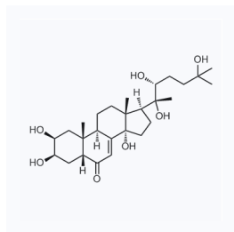
1034752 现货 CAS: 5289-74-7
