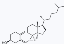
1182110 CAS: 89231-90-3
