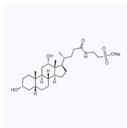
1064059 CAS: 1180-95-6
