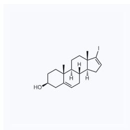
1059048 现货 CAS: 32138-69-5
