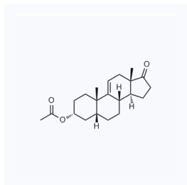
1164731 CAS: 104534-37-4
