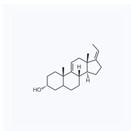
1164724 CAS: 1093397-66-0
