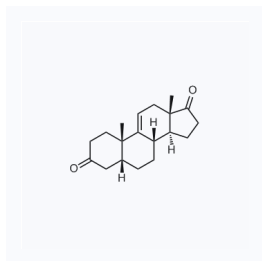
1164722 CAS: 1093397-63-7
