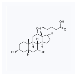
1044143 现货 CAS: 81-25-4
