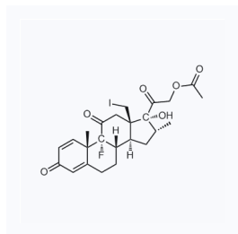
1134587 CAS: 1881-17-0
