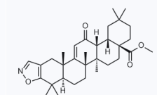
1057714 CAS: 218600-52-3
