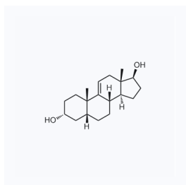
1164729 CAS: 907571-63-5
