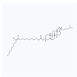
1023527 CAS: 17110-51-9
