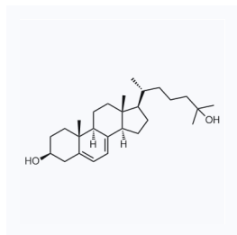
1076648 现货 CAS: 22145-68-2
