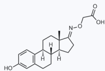
1170412 CAS: 693227-00-8
