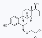
1188920 CAS: 35048-47-6
