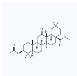
1057709 现货 CAS: 25493-94-1
