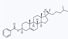
1037337 CAS: 604-32-0
