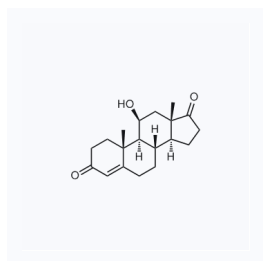
1031358 CAS: 382-44-5
