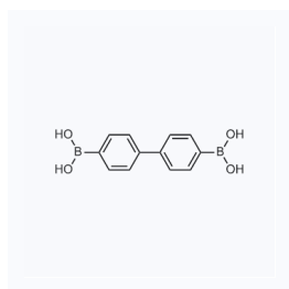
1050758 现货 CAS: 4151-80-8
