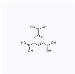
1181933 现货 CAS: 89641-21-4
