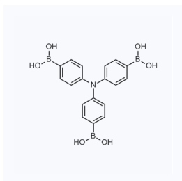
1216940 CAS: 245737-33-1
