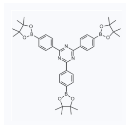
1167765 现货 CAS: 1447947-87-6
