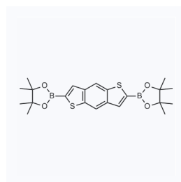
1181943 CAS: 861398-06-3
