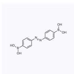
1181826 CAS: 1902168-17-5
