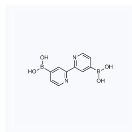
1180922 CAS: 159614-36-5
