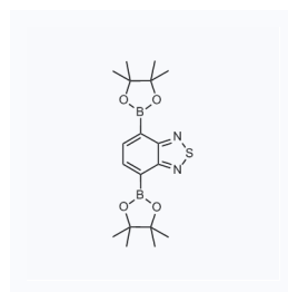
1053514 现货 CAS: 934365-16-9
