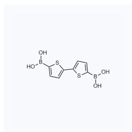
1180928 CAS: 189358-30-3
