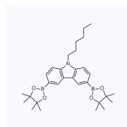
1181509 CAS: 628336-95-8
