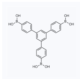
1181979 现货 CAS: 900795-73-5
