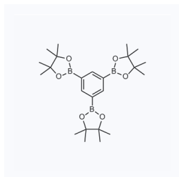
1175218 现货 CAS: 365564-05-2
