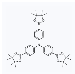
1181769 现货 CAS: 267221-90-9
