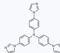
1181774 CAS: 1258947-79-3
