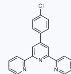
1092547 CAS: 89972-75-8
