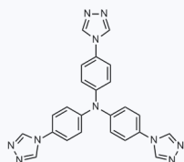
1181764 CAS: 2001066-82-4
