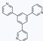
1181017 CAS: 872277-48-0
