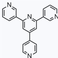
1202850 CAS: 887917-75-1
