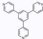
1181018 CAS: 170165-84-1
