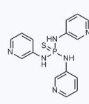
1181952 CAS: 2146095-56-7
