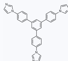
1180943 CAS: 1386857-85-7
