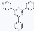
1092541 CAS: 42333-78-8
