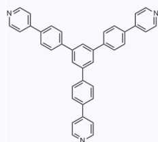
1181955 CAS: 170165-85-2
