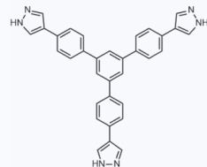
1181846 CAS: 1855846-73-9
