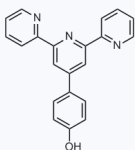
1216907 CAS: 89972-79-2
