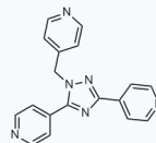
1181929 CAS: 55391-42-9
