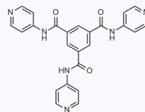
1181484 CAS: 725274-03-3
