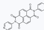
1169555 CAS: 34151-49-0
