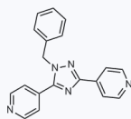
1181948 CAS: 55391-37-2
