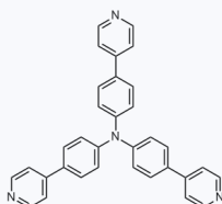
1181762 CAS: 1366291-62-4
