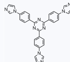
1202776 CAS: 1009564-95-7
