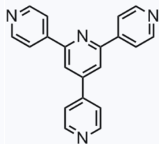
1202784 CAS: 113919-79-2
