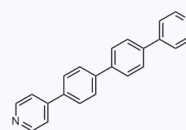
1181418 CAS: 319430-87-0
