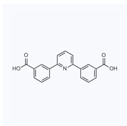
1181440 CAS: 1258419-69-0
