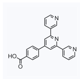
1202832 CAS: 1415258-35-3
