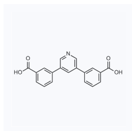
1181442 CAS: 1429436-06-5
