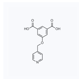
1181478 CAS: 1240327-15-4
