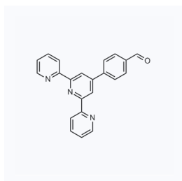
1181548 CAS: 138253-30-2
