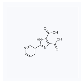
1181096 CAS: 51294-28-1
