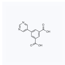
1181091 CAS: 1417570-15-0
