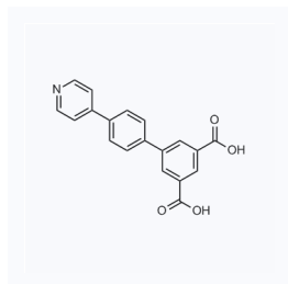
1181251 现货 CAS: 2022152-71-0
