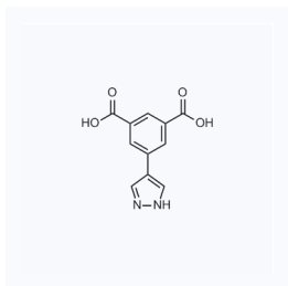
1181426 现货 CAS: 1108726-74-4
