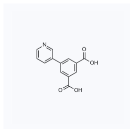
1181127 CAS: 1264068-70-3
