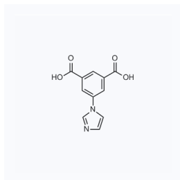
1181421 CAS: 1643586-52-0
