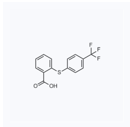
1216804 CAS: 895-45-4
