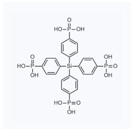
1181913 CAS: 1808003-51-1
