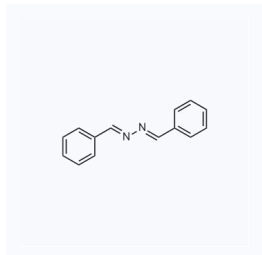
1216811 CAS: 28867-76-7
