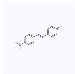
1216818 CAS: 48174-78-3
