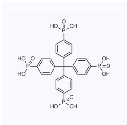
1182071 CAS: 1632402-15-3
