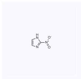
1034723 CAS: 527-73-1
