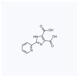
1181095 CAS: 1025042-44-7
