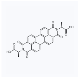
1181894 CAS: 925685-87-6
