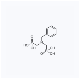
1180812 CAS: 6056-53-7
