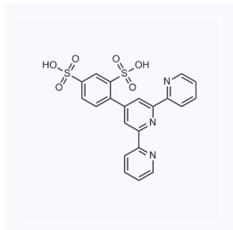
1181056 CAS: 1458013-19-8
