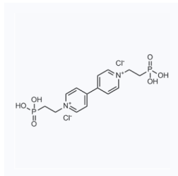
1181822 CAS: 151538-79-3
