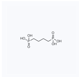
1182085 CAS: 4671-77-6
