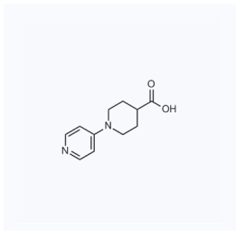
1180942 CAS: 93913-86-1
