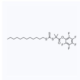
1204054 CAS: 1174764-26-1
