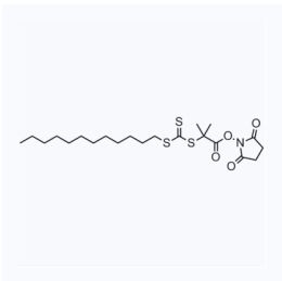
1204055 CAS: 925232-64-0
