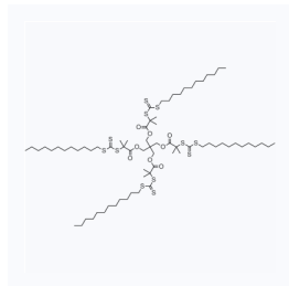
1204033 CAS: 1435934-76-1
