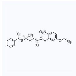
1204010 CAS: 1318075-32-9
