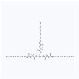
1204028 CAS: 1435934-51-2
