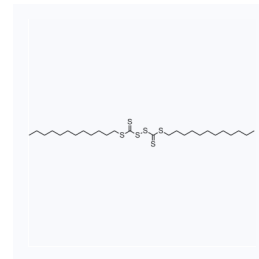
1203993 CAS: 870532-86-8
