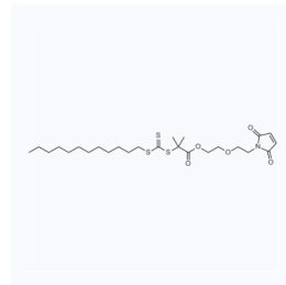
1172385 CAS: 1050217-24-7
