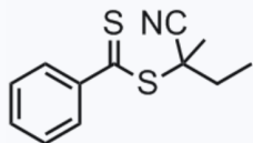
1203990 CAS: 220182-83-2
