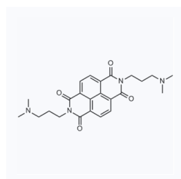
1169543 CAS: 3436-54-2
