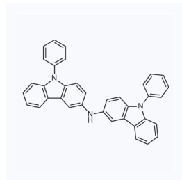
1216962 CAS: 1933473-91-6
