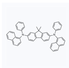
1216992 CAS: 222319-05-3
