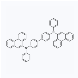
1216955 CAS: 934000-87-0
