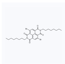
1169558 CAS: 926643-78-9
