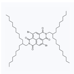
1169551 CAS: 1100243-35-3
