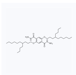
1216942 CAS: 2413366-64-8
