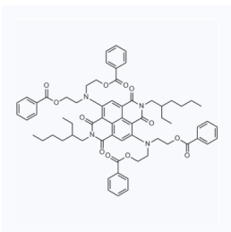
1180810 CAS: 2043039-70-7
