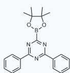
1206513 CAS: 1345345-08-5
