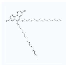
1181543 CAS: 473255-23-1
