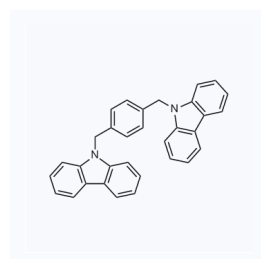
1216957 CAS: 166256-60-6
