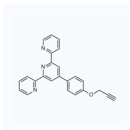
1181342 CAS: 1628933-55-0
