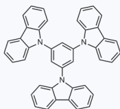
1021864 现货 CAS: 148044-07-9
