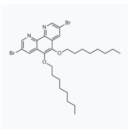
1181544 CAS: 473255-19-5
