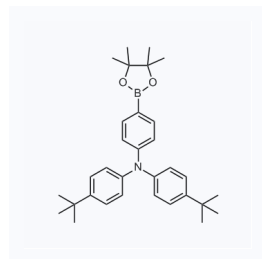
1167339 CAS: 935480-19-6
