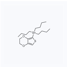
1181781 CAS: 175922-79-9
