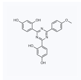
1167410 CAS: 1440-00-2
