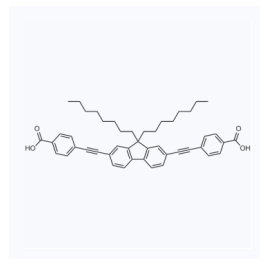
1216899 CAS: 1313187-39-1
