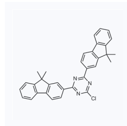
1206503 CAS: 1459162-69-6
