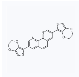
1181541 CAS: 1001330-07-9
