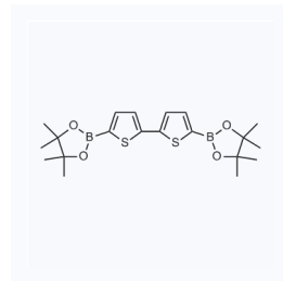
1162294 CAS: 239075-02-6
