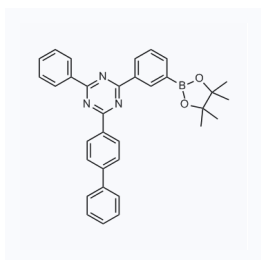
1206510 CAS: 1696425-30-5
