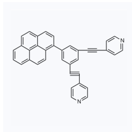
1181987 CAS: 2097132-49-3
