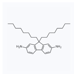
1169559 CAS: 851042-10-9
