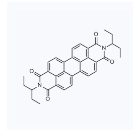
1181400 CAS: 110590-81-3
