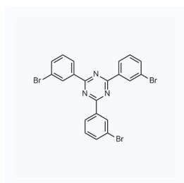
1169446 CAS: 890148-78-4
