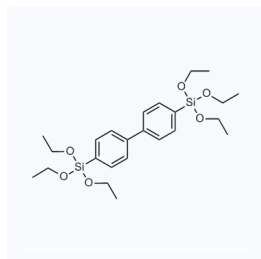
1216970 CAS: 123640-93-7
