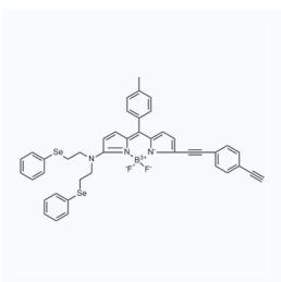
1182193 CAS: 1962170-57-5
