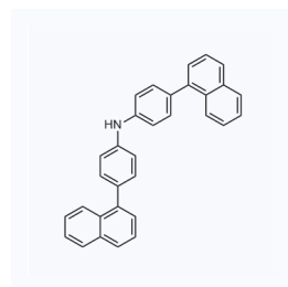
1216988 CAS: 897671-74-8
