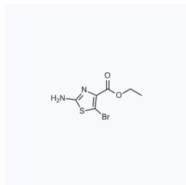
1069428 现货 CAS: 61830-21-5
