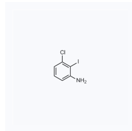
1062600 现货 CAS: 70237-25-1
