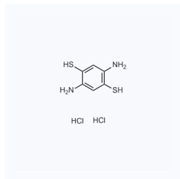
1042042 现货 CAS: 75464-52-7
