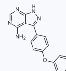
1060227 CAS: 330786-24-8
