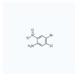
1063514 现货 CAS: 827-33-8
