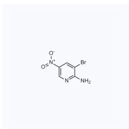
1052010 现货 CAS: 15862-31-4
