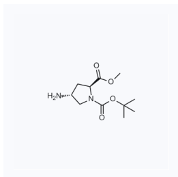
1059513 现货 CAS: 121148-00-3
