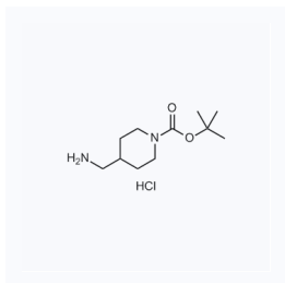
1065344 现货 CAS: 359629-16-6
