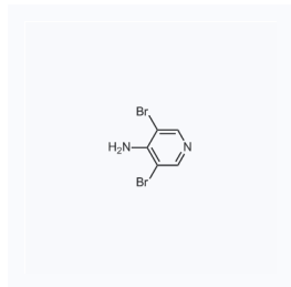
1044619 现货 CAS: 84539-34-4
