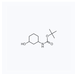
1037554 现货 CAS: 610302-03-9
