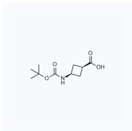
1069386 现货 CAS: 1008773-79-2
