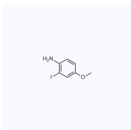
1062333 现货 CAS: 191348-14-8
