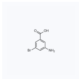
1032463 现货 CAS: 42237-85-4
