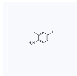
1059483 现货 CAS: 4102-53-8
