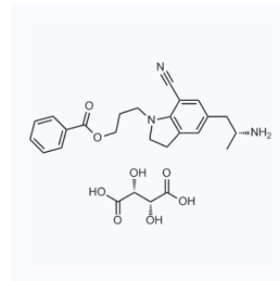
1057674 现货 CAS: 239463-85-5
