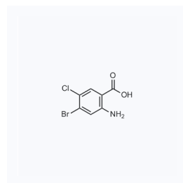
1064685 现货 CAS: 150812-32-1
