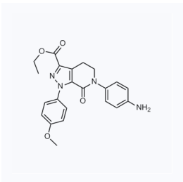
1058756 现货 CAS: 503615-07-4
