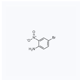
1045453 现货 CAS: 875-51-4
