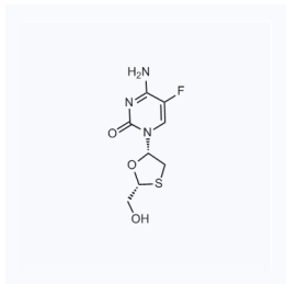
1021411 现货 CAS: 143491-57-0
