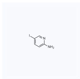
1025369 现货 CAS: 20511-12-0
