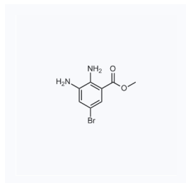
1067138 现货 CAS: 1248541-63-0
