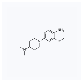
1117323 现货 CAS: 1089279-91-3
