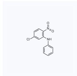
1027551 现货 CAS: 25781-92-4
