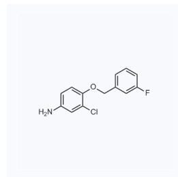
1068537 现货 CAS: 202197-26-0
