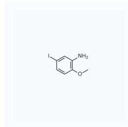
1043046 现货 CAS: 77770-09-3
