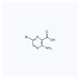
1062814 现货 CAS: 486424-37-7
