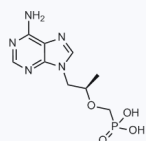
1021791 CAS: 147127-20-6
