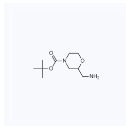
1052413 现货 CAS: 140645-53-0
