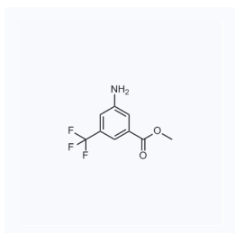
1063995 现货 CAS: 22235-25-2
