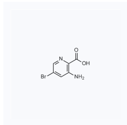
1045274 现货 CAS: 870997-85-6
