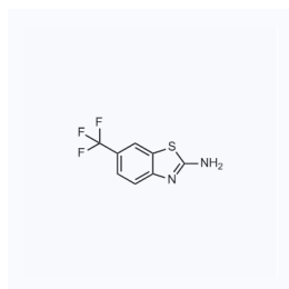
1107652 现货 CAS: 777-12-8
