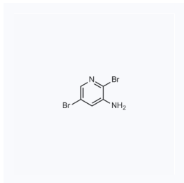
1122783 现货 CAS: 90902-84-4
