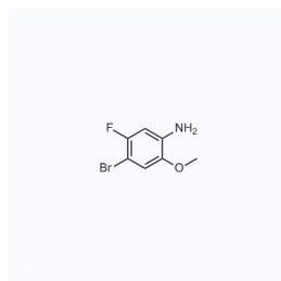
1066262 现货 CAS: 330794-03-1
