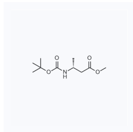
1074016 现货 CAS: 159877-47-1
