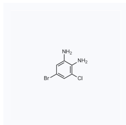
1167653 现货 CAS: 16429-44-0
