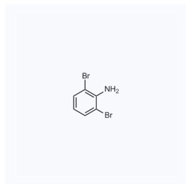
1037484 现货 CAS: 608-30-0
