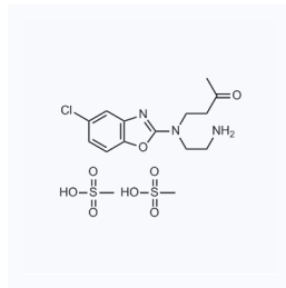
1057647 现货 CAS: 1276666-12-6
