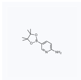
1044374 现货 CAS: 827614-64-2
