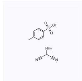
1063210 现货 CAS: 5098-14-6
