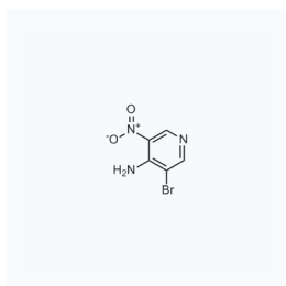
1064707 现货 CAS: 89284-05-9
