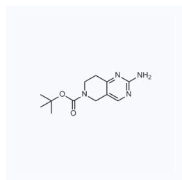
1063268 现货 CAS: 869198-95-8
