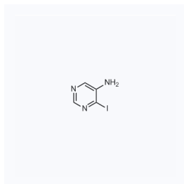
1063888 现货 CAS: 942067-98-3
