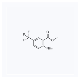
1065467 现货 CAS: 117324-58-0
