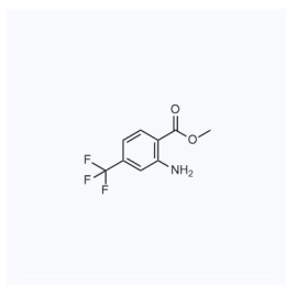
1069595 现货 CAS: 61500-87-6
