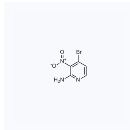
1064500 现货 CAS: 84487-10-5
