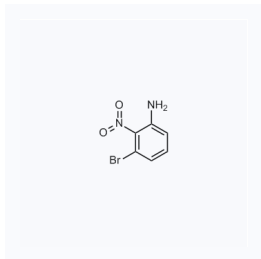
1040626 现货 CAS: 7138-15-0
