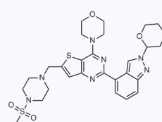
1057536 CAS: 1146955-37-4
