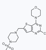
1058257 CAS: 885675-66-1
