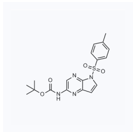
1118596 CAS: 1201187-44-1
