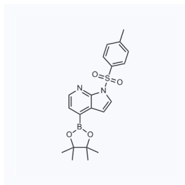
1051408 CAS: 916176-50-6
