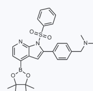
1058374 现货 CAS: 942919-72-4
