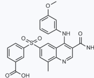
1058699 CAS: 801311-41-1
