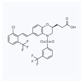
1122224 CAS: 1807791-77-0
