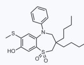
1160683 CAS: 439088-16-1
