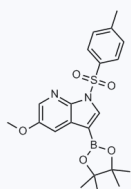
1121088 CAS: 1355221-17-8
