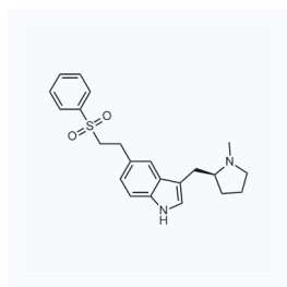
1057144 CAS: 1252673-29-2
