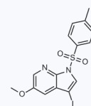
1075140 CAS: 945256-30-4
