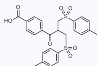
1176960 CAS: 124243-00-1
