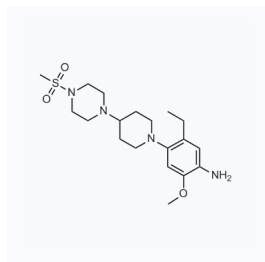
1057281 CAS: 1089282-91-6
