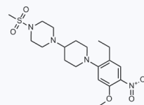
1057280 CAS: 1089282-90-5
