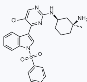
1185018 CAS: 1816989-75-9
