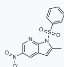
1075019 CAS: 1186501-88-1
