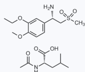
1060490 现货 CAS: 608141-43-1
