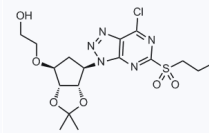
1060064 现货 CAS: 1863036-47-8
