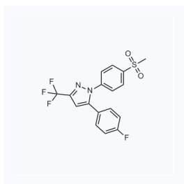
1022924 CAS: 162054-19-5
