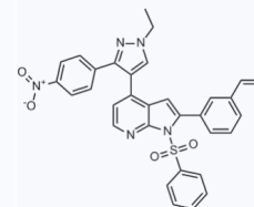
1058515 CAS: 942920-00-5
