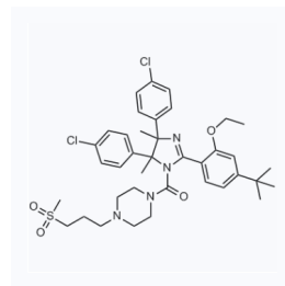
1077051 CAS: 1313611-29-8
