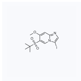
1139570 CAS: 2141961-59-1
