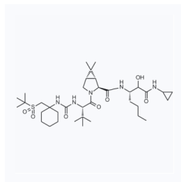
1057624 CAS: 1208245-90-2
