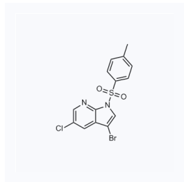
1074285 CAS: 866546-10-3
