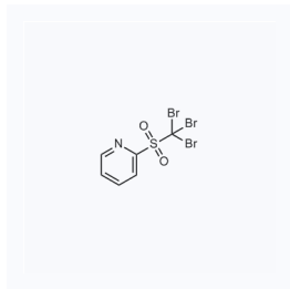
1037046 CAS: 59626-33-4
