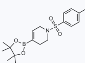
1067193 现货 CAS: 1256360-46-9
