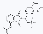
1066756 现货 CAS: 253168-86-4
