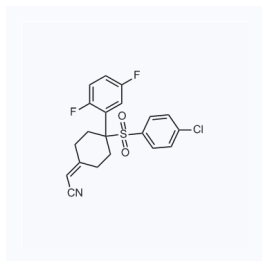
1057249 CAS: 656810-84-3
