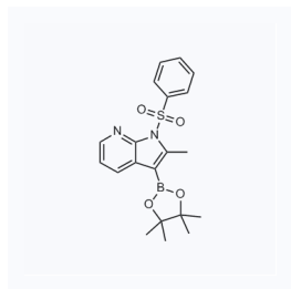
1074273 CAS: 943324-08-1
