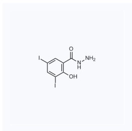
1141173 CAS: 89011-15-4
