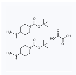
1118855 CAS: 1818847-34-5
