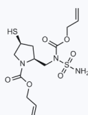
1057009 CAS: 148017-51-0
