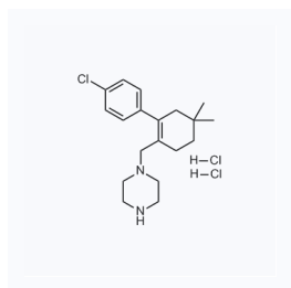
1066782 现货 CAS: 1628047-87-9
