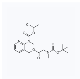
1061984 现货 CAS: 338990-31-1
