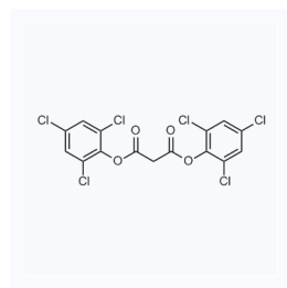
1062930 现货 CAS: 15781-70-1
