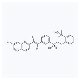
1021270 现货 CAS: 142569-70-8
