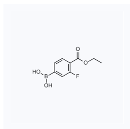
1045401 现货 CAS: 874288-38-7
