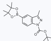
1156007 现货 CAS: 864770-82-1
