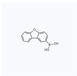
1111065 现货 CAS: 402936-15-6
