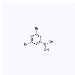
1164411 现货 CAS: 2096340-19-9
