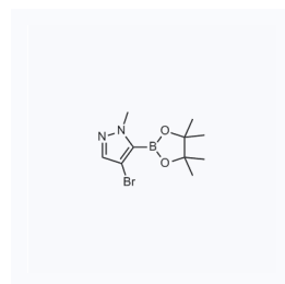
1111791 现货 CAS: 942070-88-4
