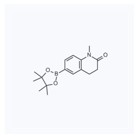
1125497 现货 CAS: 1427587-32-3
