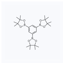
1175218 CAS: 365564-05-2
