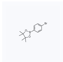
1106688 现货 CAS: 68716-49-4
