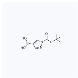
1063305 现货 CAS: 1188405-87-9
