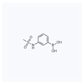
1182961 现货 CAS: 148355-75-3
