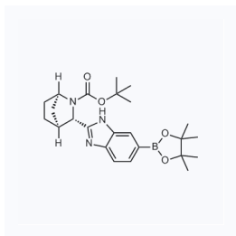
1060329 CAS: 1256387-87-7
