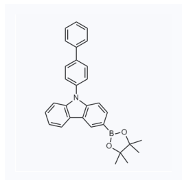
1162280 CAS: 1391729-66-0
