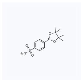
1183505 现货 CAS: 214360-51-7
