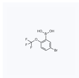
1109621 现货 CAS: 1072951-56-4
