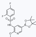
1058506 现货 CAS: 1083326-73-1
