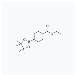
1064438 现货 CAS: 1049004-32-1
