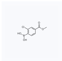
1062978 现货 CAS: 603122-80-1
