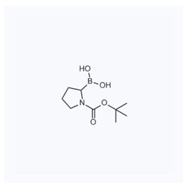
1061576 现货 CAS: 149682-75-7
