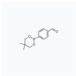
1201042 现货 CAS: 128376-65-8
