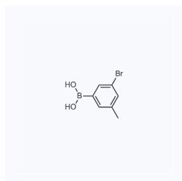
1050787 现货 CAS: 849062-36-8
