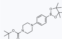
1059888 现货 CAS: 470478-90-1
