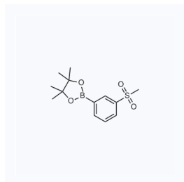
1109939 现货 CAS: 1001185-88-1
