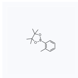
1050733 现货 CAS: 195062-59-0
