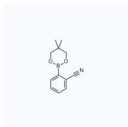
1050737 现货 CAS: 214360-47-1
