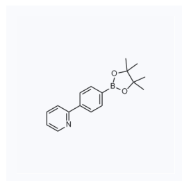
1111826 现货 CAS: 908350-80-1
