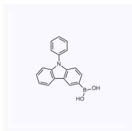
1067180 现货 CAS: 854952-58-2
