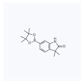
1172779 现货 CAS: 1190861-74-5
