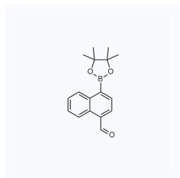
1084254 现货 CAS: 1008361-71-4
