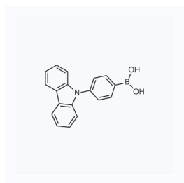
1050759 现货 CAS: 419536-33-7
