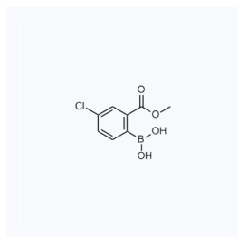
1132451 现货 CAS: 1612256-37-7
