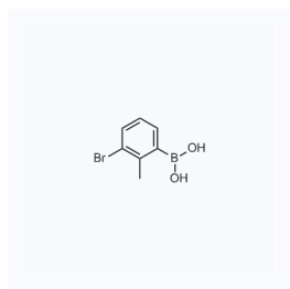
1169780 现货 CAS: 1184298-27-8
