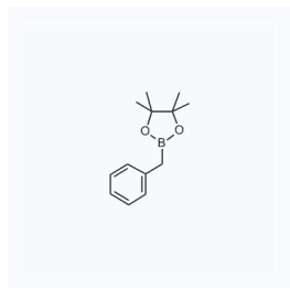
1045275 现货 CAS: 87100-28-5
