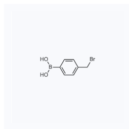
1039786 现货 CAS: 68162-47-0
