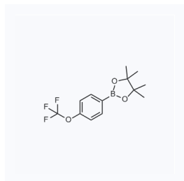
1151788 现货 CAS: 474709-28-9
