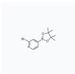
1033038 现货 CAS: 458532-82-6
