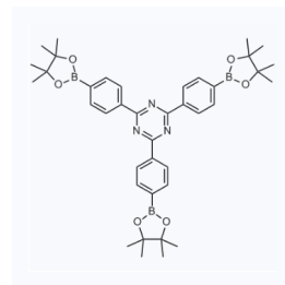
1167765 CAS: 1447947-87-6
