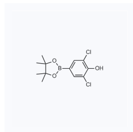
1059602 现货 CAS: 1003298-87-0
