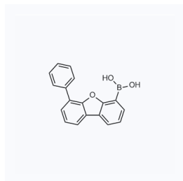
1061457 现货 CAS: 1010068-85-5
