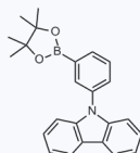
1165952 现货 CAS: 870119-58-7
