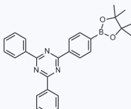
1165961 现货 CAS: 1219956-23-6
