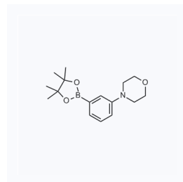
1063045 现货 CAS: 852227-95-3
