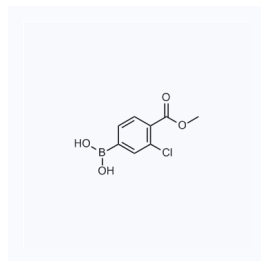
1052449 现货 CAS: 603122-82-3
