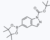
1069952 现货 CAS: 864771-44-8
