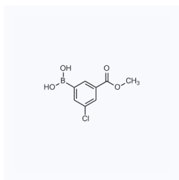
1170454 现货 CAS: 957120-26-2
