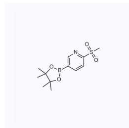
1122863 现货 CAS: 1052138-94-9
