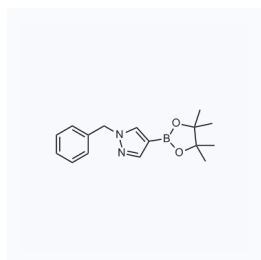
1042277 现货 CAS: 761446-45-1
