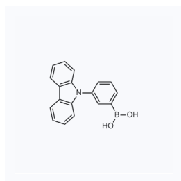
1053048 现货 CAS: 864377-33-3
