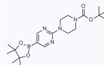
1069965 现货 CAS: 940284-98-0
