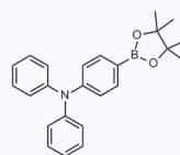
1201117 现货 CAS: 267221-88-5
