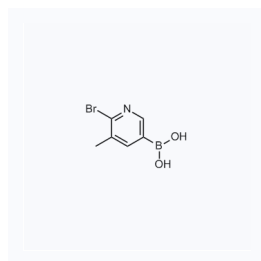
1014606 现货 CAS: 1003043-34-2
