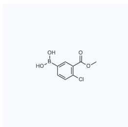
1063082 现货 CAS: 874219-45-1
