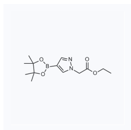
1045086 现货 CAS: 864754-16-5
