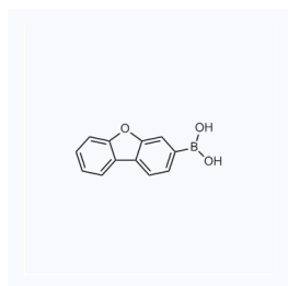
1165958 现货 CAS: 395087-89-5
