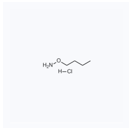
1176820 现货 CAS: 4490-82-8
