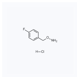
1114332 现货 CAS: 51572-89-5
