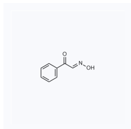
1034873 现货 CAS: 532-54-7
