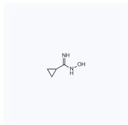
1062708 现货 CAS: 51285-13-3
