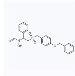
1193011 CAS: 1253527-86-4
