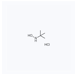
1200909 现货 CAS: 57497-39-9
