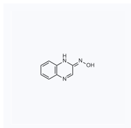
1203405 现货 CAS: 41443-27-0
