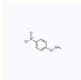
1069740 现货 CAS: 33543-55-4
