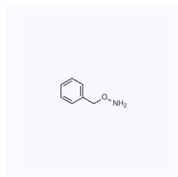
1062403 现货 CAS: 622-33-3
