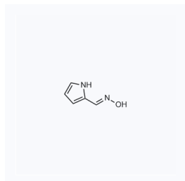
1107176 现货 CAS: 32597-34-5
