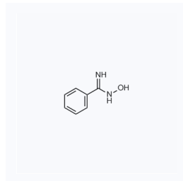
1037727 现货 CAS: 613-92-3
