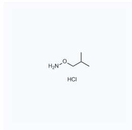
1206654 现货 CAS: 6084-58-8
