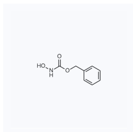
1190658 现货 CAS: 3426-71-9
