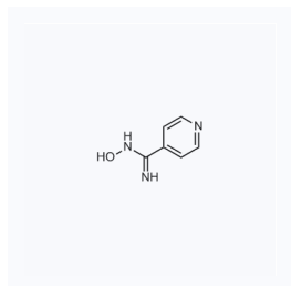
1130906 现货 CAS: 1594-57-6
