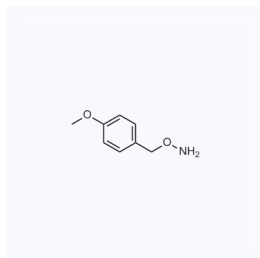
1053483 现货 CAS: 21038-22-2
