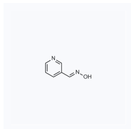
1203033 现货 CAS: 1193-92-6
