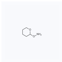
1039524 现货 CAS: 6723-30-4
