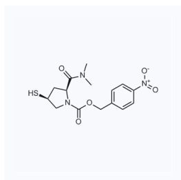
1063872 CAS: 96034-64-9
