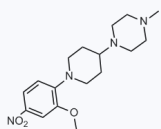
1061223 现货 CAS: 1254058-33-7
