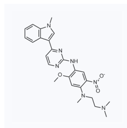
1060380 CAS: 1421372-67-9
