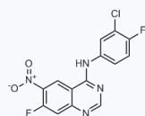
1057256 现货 CAS: 162012-67-1
