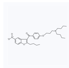
1058590 CAS: 141645-23-0
