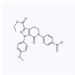
1058755 CAS: 536759-91-8
