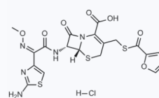
1015500 CAS: 103980-44-5
