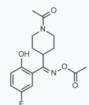
1203517 CAS: 84163-52-0
