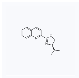
1175076 现货 CAS: 933992-49-5
