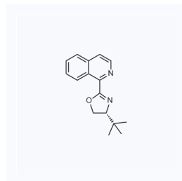
1158560 现货 CAS: 1402851-53-9
