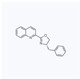
1158490 现货 CAS: 1252576-14-9
