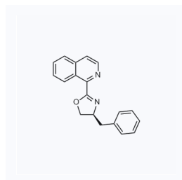
1215742 现货 CAS: 2058236-52-3
