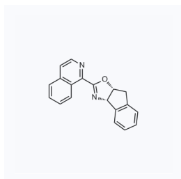
1215746 现货 CAS: 2222863-66-1
