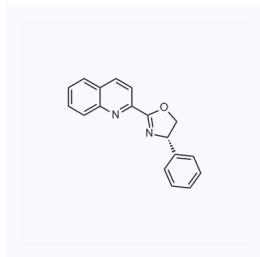
1158935 现货 CAS: 1252576-13-8
