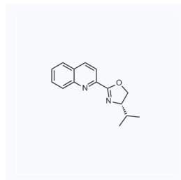
1158504 现货 CAS: 226387-11-7
