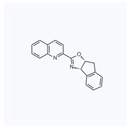
1167441 现货 CAS: 2055935-90-3
