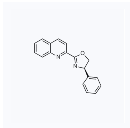
1167440 现货 CAS: 220108-54-3
