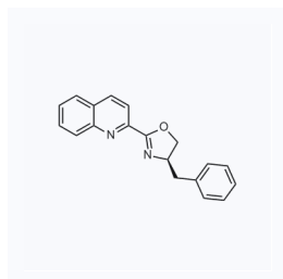
1175075 现货 CAS: 933992-48-4
