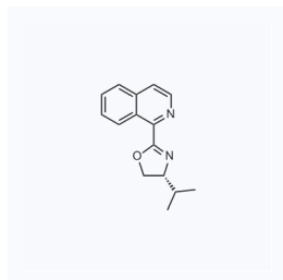
1158179 现货 CAS: 280755-83-1
