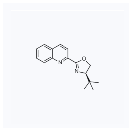
1175078 现货 CAS: 1402851-53-9
