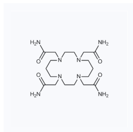
1158048 CAS: 345612-63-7
