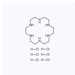
1155720 CAS: 58105-91-2
