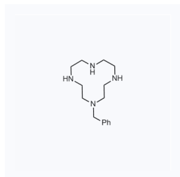
1176327 CAS: 112193-83-6
