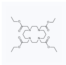
1091932 CAS: 126320-57-8
