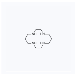
1028604 CAS: 295-37-4
