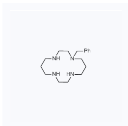
1176866 CAS: 132723-93-4
