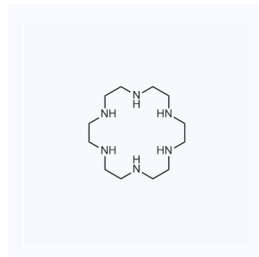
1156486 CAS: 296-35-5
