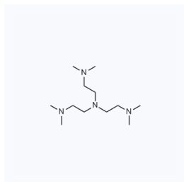
1029974 CAS: 33527-91-2
