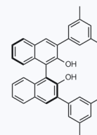
1157436 CAS: 435327-17-6
