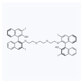
1163973 CAS: 1260243-73-9
