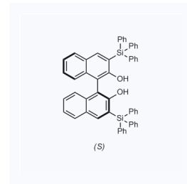
1157178 CAS: 111795-33-6
