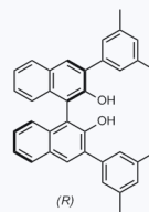
1157596 CAS: 215433-51-5
