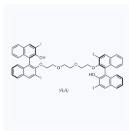
1163972 CAS: 1411975-49-9
