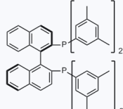
1020658 CAS: 137219-86-4
