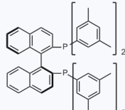
1020424 CAS: 135139-00-3
