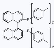
1014512 CAS: 100165-88-6
