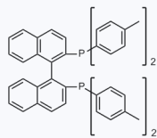
1180562 CAS: 153305-67-0
