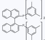
1157153 CAS: 145416-77-9
