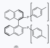
1047825 CAS: 99646-28-3
