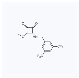
1169121 CAS: 1073917-05-1
