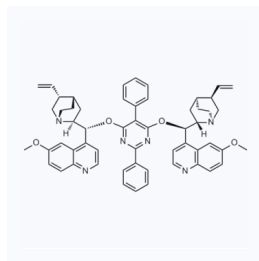
1164250 CAS: 189745-70-8
