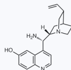
1175609 CAS: 960050-59-3
