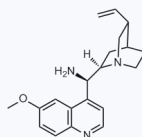
1161536 CAS: 287979-82-2
