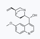
1171467 CAS: 572-59-8
