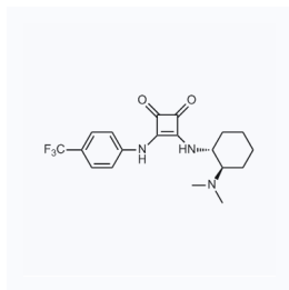
1163877 CAS: 1565829-15-3
