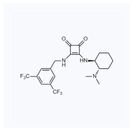
1163879 CAS: 1570357-02-6
