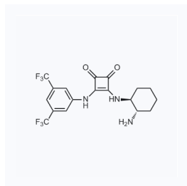
1174955 CAS: 1312991-12-0
