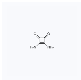
1117343 CAS: 5231-89-0
