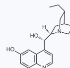
1164256 CAS: 73522-75-5
