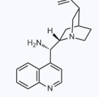
1175597 CAS: 1263486-03-8
