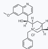
1042856 CAS: 77481-82-4
