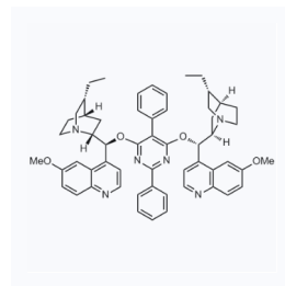
1022035 CAS: 149725-81-5
