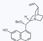
1164251 CAS: 761434-35-9
