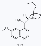
1175599 CAS: 931098-91-8
