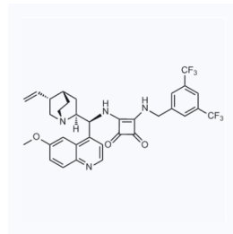
1163578 现货 CAS: 1210360-60-3
