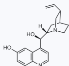
1164253 CAS: 524-63-0
