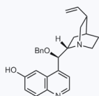
1175602 CAS: 838821-39-9
