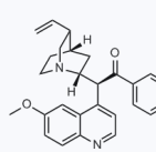
1162073 CAS: 60723-45-7
