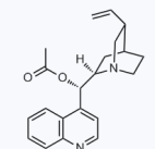
1163857 CAS: 14461-05-3
