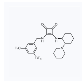
1163880 CAS: 1570357-03-7
