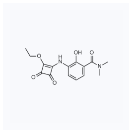
1057164 CAS: 464913-33-5
