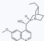
1021425 现货 CAS: 1435-55-8
