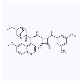
1163838 现货 CAS: 1407166-63-5
