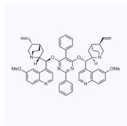
1175592 CAS: 1202521-49-0
