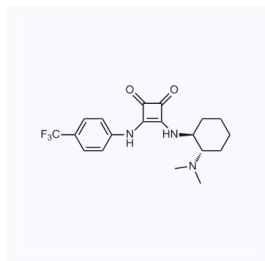
1163724 CAS: 1312991-14-2
