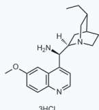
1175598 CAS: 931098-92-9
