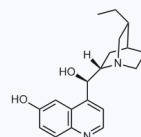
1175605 CAS: 5962-19-6
