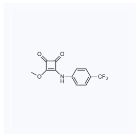
1169125 CAS: 1132827-67-8
