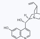
1164255 CAS: 70877-75-7
