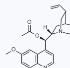
1161460 CAS: 18797-86-9
