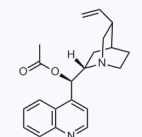
1163840 CAS: 14075-54-8
