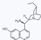
1175610 CAS: 1430820-98-6
