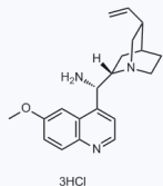
1175594 现货 CAS: 1231763-32-8
