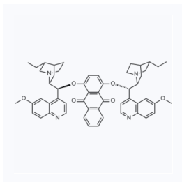
1163953 CAS: 176298-44-5
