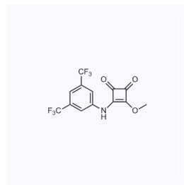
1169115 CAS: 1223105-85-8
