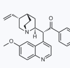
1162115 CAS: 69758-70-9
