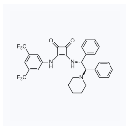
1164249 现货 CAS: 1454257-32-9
