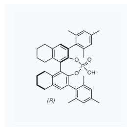
1163352 CAS: 1011465-23-8
