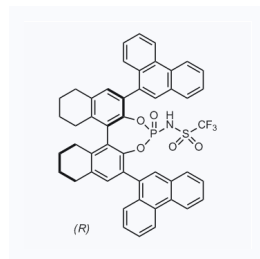
1163553 现货 CAS: 1181834-74-1
