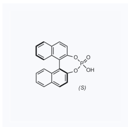
1030538 现货 CAS: 35193-64-7
