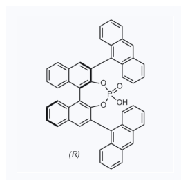
1070018 现货 CAS: 361342-51-0
