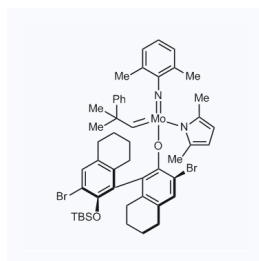
1182473 CAS: 1300026-28-1
