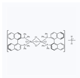
1025068 CAS: 199684-47-4
