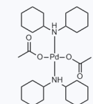
1038324 CAS: 628339-96-8
