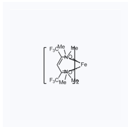
1181805 CAS: 73450-43-8
