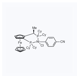
1181324 CAS: 2049086-35-1
