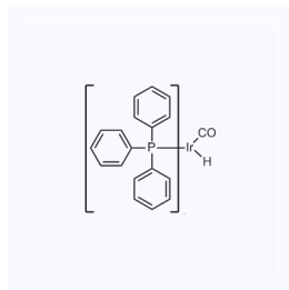
1153231 CAS: 17250-25-8
