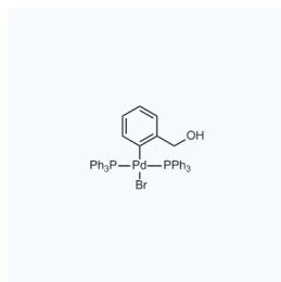
1179791 CAS: 849417-41-0
