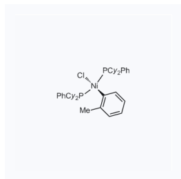
1156002 CAS: 1419179-26-2
