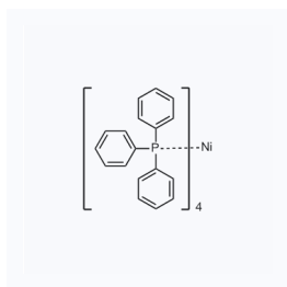
1112938 CAS: 15133-82-1
