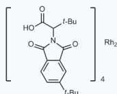
1202636 CAS: 1884452-99-6
