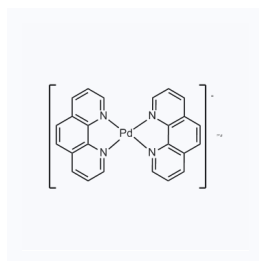
1151476 CAS: 113173-22-1
