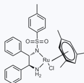
1151705 CAS: 174813-81-1
