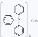
1022623 现货 CAS: 15709-74-7
