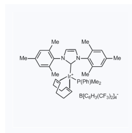
1153551 CAS: 1884137-92-1
