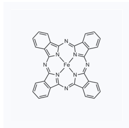
1176627 CAS: 132-16-1
