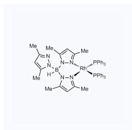
1180800 CAS: 341483-76-9
