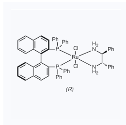
1025773 CAS: 212210-87-2
