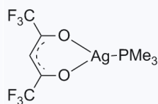
1181907 CAS: 148630-66-4
