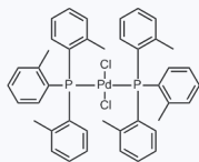
1091997 现货 CAS: 40691-33-6
