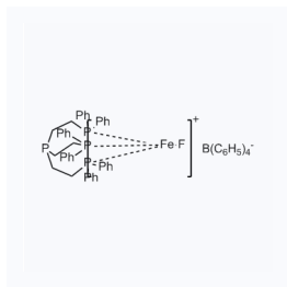
1181877 CAS: 1318882-57-3
