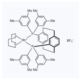
1180786 CAS: 619334-93-9
