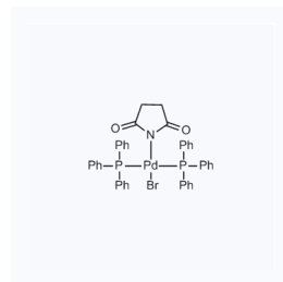
1027319 CAS: 251567-28-9
