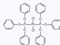
1028754 CAS: 30053-58-8
