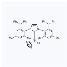
1181399 CAS: 1955555-28-8
