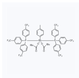
1044861 CAS: 851530-57-9
