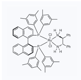
1026125 CAS: 220114-03-4
