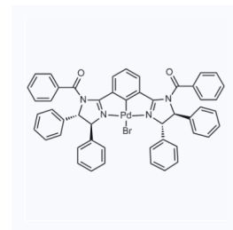
1151529 CAS: 1242081-29-3
