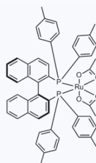
1151721 CAS: 106681-15-6
