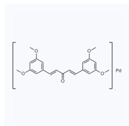
1044131 CAS: 811862-77-8
