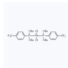
1045724 CAS: 887919-36-0
