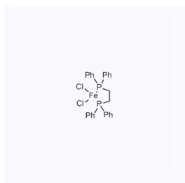
1181811 CAS: 41536-18-9
