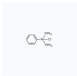
1181463 CAS: 33571-43-6
