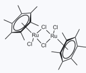
1152722 CAS: 67421-02-7
