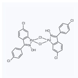
1151388 CAS: 287410-78-0
