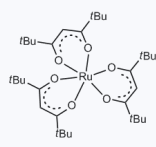
1155322 CAS: 38625-54-6
