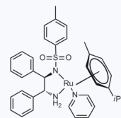
1154849 CAS: 1192483-14-9
