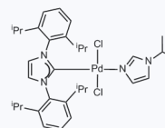
1161583 CAS: 1537172-99-8
