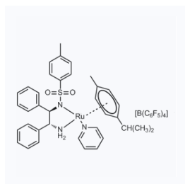
1154887 CAS: 1192483-19-4
