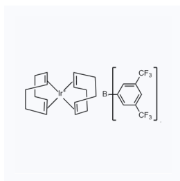
1153345 CAS: 666826-16-0
