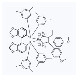
1152738 CAS: 944450-43-5
