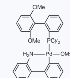
1151412 现货 CAS: 1445085-82-4
