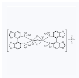
1155670 CAS: 944451-14-3
