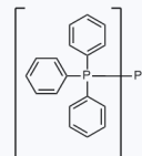
1021232 现货 CAS: 14221-01-3
