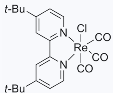
1182418 CAS: 165612-19-1
