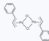
1105805 现货 CAS: 12131-44-1
