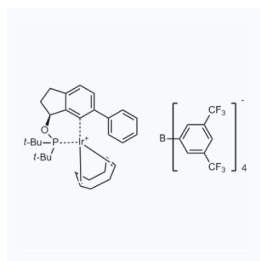
1181233 CAS: 881310-39-0
