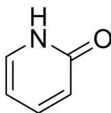
Pyridin-2(1H)-one
