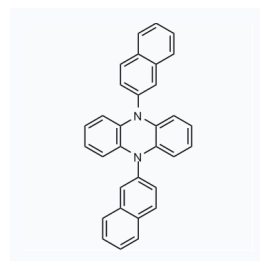
1176306 CAS: 1934269-97-2
