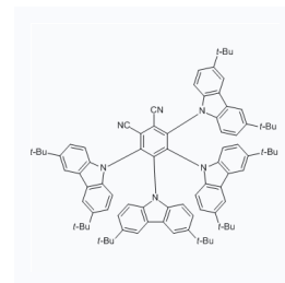
1175932 现货 CAS: 1469705-93-8
