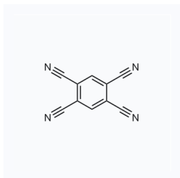
1040600 现货 CAS: 712-74-3
