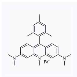
1284510 CAS: 2180894-90-8
