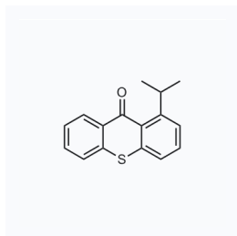
1035573 现货 CAS: 5495-84-1
