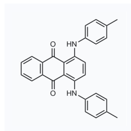
1135110 现货 CAS: 128-80-3
