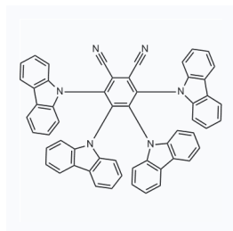
1176318 现货 CAS: 1416881-51-0
