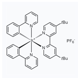
1153235 现货 CAS: 676525-77-2
