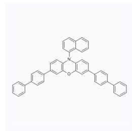
1176301 CAS: 1987900-95-7
