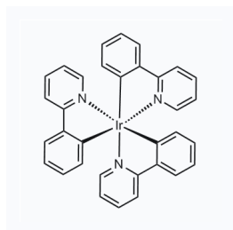
1047180 现货 CAS: 94928-86-6
