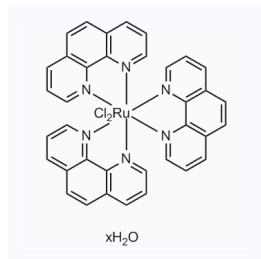
1155307 现货 CAS: 207802-45-7
