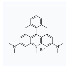
1284518 CAS: 2380163-04-0
