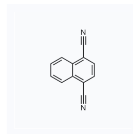
1212833 CAS: 3029-30-9
