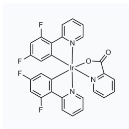
1031216 现货 CAS: 376367-93-0
