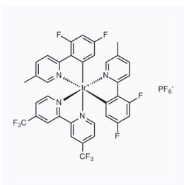
1237558 现货 CAS: 2229858-27-7
