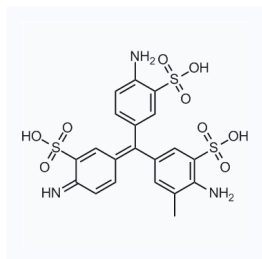
1284505 CAS: 19379-19-2
