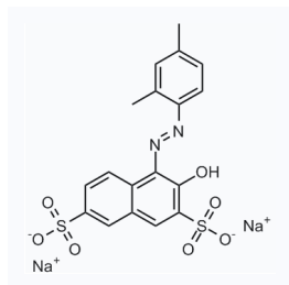
1178288 CAS: 3761-53-3
