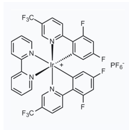
1153401 现货 CAS: 1092775-62-6
