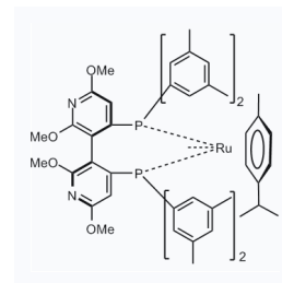
1284459 CAS: 1034001-49-4
