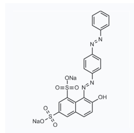
1208879 CAS: 5413-75-2
