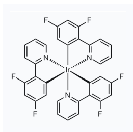
1153402 现货 CAS: 387859-70-3
