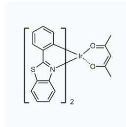
1181213 CAS: 337526-88-2
