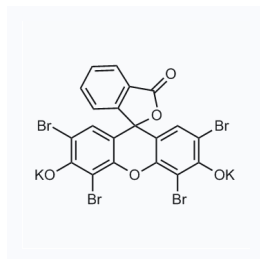
1271983 CAS: 56897-54-2
