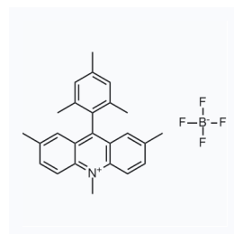
1176208 现货 CAS: 1621019-97-3
