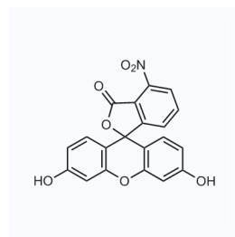
1284472 CAS: 3318-08-9
