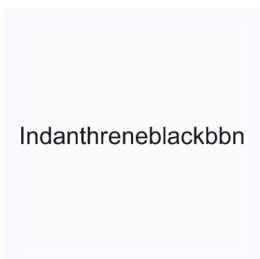
1284461 CAS: 6369-65-9
