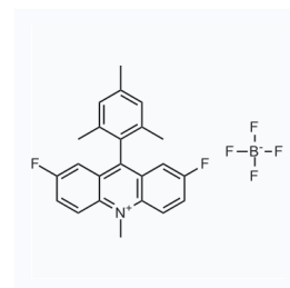
1176167 现货 CAS: 2635339-88-5
