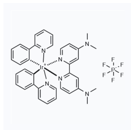
1597622 CAS: 918890-29-6
