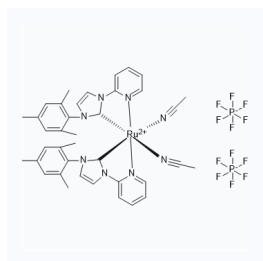
1597628 CAS: 2088512-45-0
