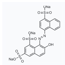
1085994 现货 CAS: 2611-82-7
