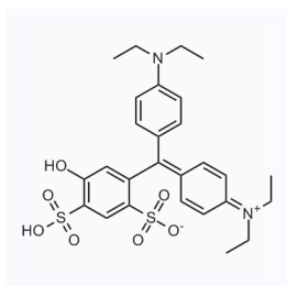
1284502 CAS: 25305-77-5
