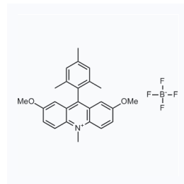
1175916 现货 CAS: 2635339-81-8
