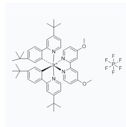
1597618 CAS: 1567403-07-9
