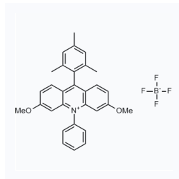
1176214 CAS: 1965330-57-7
