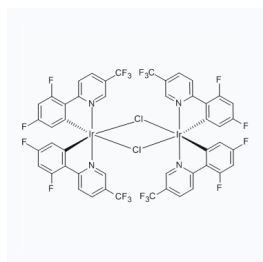
1153584 CAS: 870987-64-7
