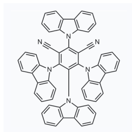
1169625 现货 CAS: 1416881-52-1
