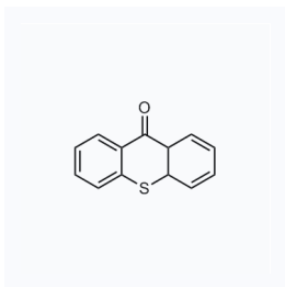
1284507 CAS: 126395-12-8
