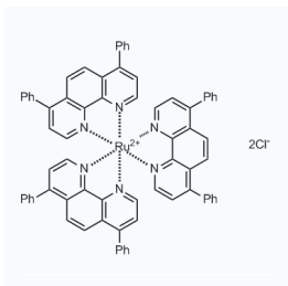
1180811 现货 CAS: 36309-88-3
