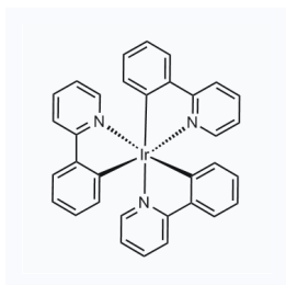
1047180 现货 CAS: 94928-86-6
