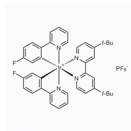
1180589 现货 CAS: 1449110-90-0
