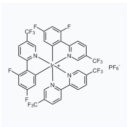
1153553 现货 CAS: 1973375-72-2
