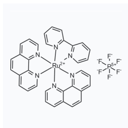
1269849 现货 CAS: 60828-39-9
