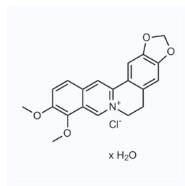
1284504 现货 CAS: 141433-60-5
