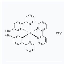
1180590 现货 CAS: 1352428-78-4
