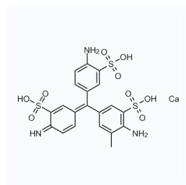
1284508 CAS: 136132-76-8
