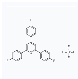
1176314 CAS: 62497-19-2
