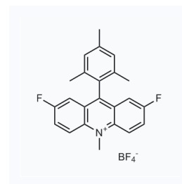
1284454 CAS: 2635339-88-5
