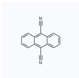
1190651 现货 CAS: 1217-45-4
