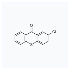
1045073 CAS: 86-39-5
