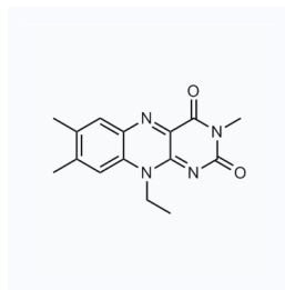
1176309 CAS: 67767-38-8
