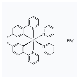
1180588 现货 CAS: 1580547-45-0
