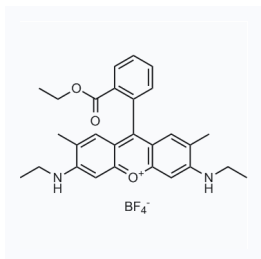
1284514 CAS: 54854-14-7
