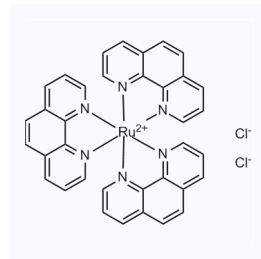
1284496 CAS: 23570-43-6
