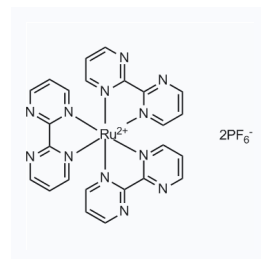
1269918 现货 CAS: 85335-55-3
