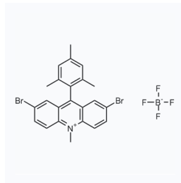
1175914 CAS: 2635339-83-0
