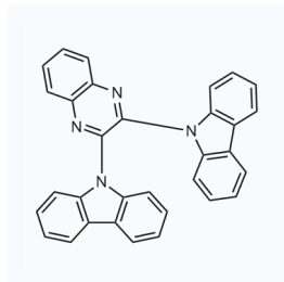
1509511 CAS: 2189730-32-1
