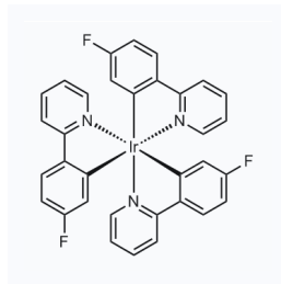
1153490 CAS: 370878-69-6
