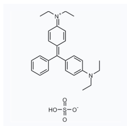
1239698 现货 CAS: 633-03-4
