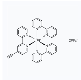
1180807 现货 CAS: 164357-77-1
