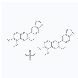
1029329 现货 CAS: 316-41-6
