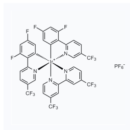
1181216 现货 CAS: 2030437-90-0
