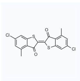
1136476 CAS: 2379-74-0
