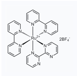
1154945 现货 CAS: 1254690-00-0
