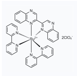
1155205 现货 CAS: 1610356-29-0
